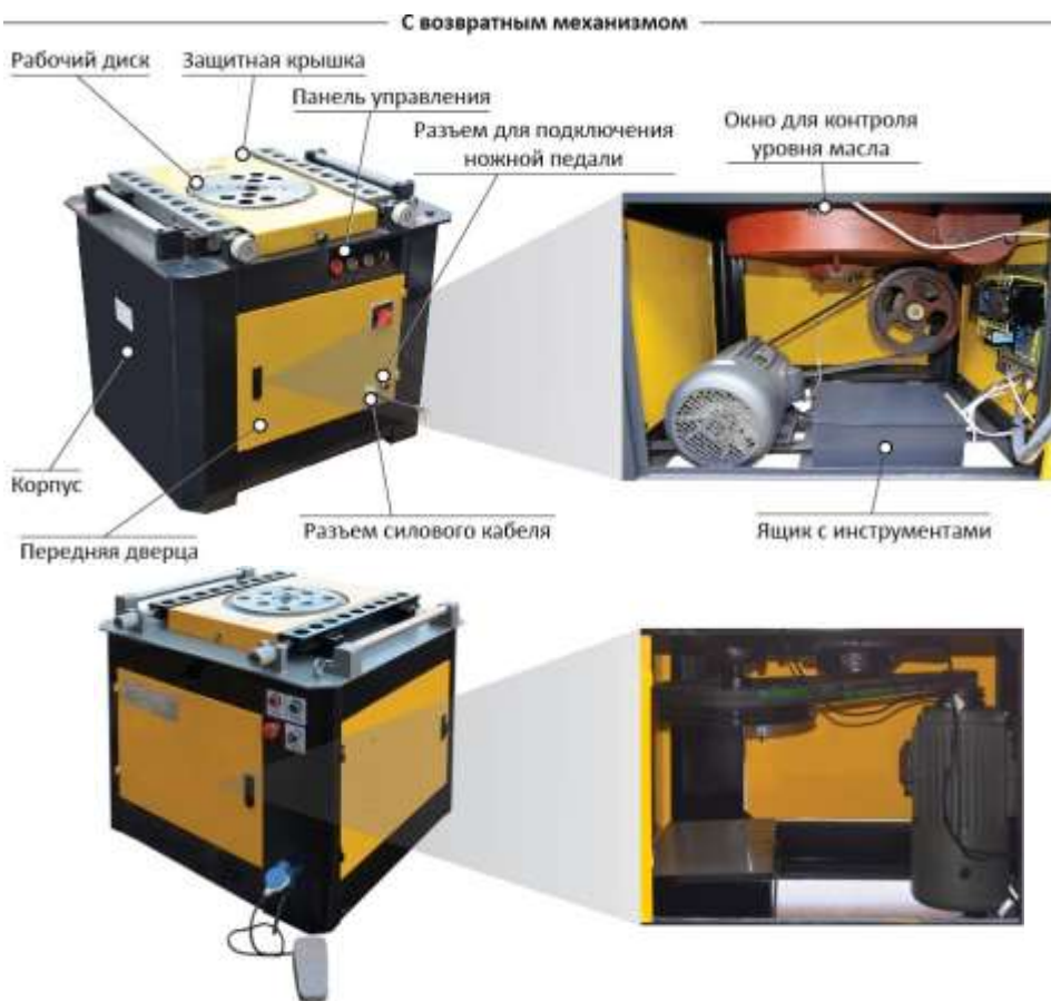
Рис. 1 - Общий вид GW40A, GW50A, GW40A-Q, GW50A-Q
