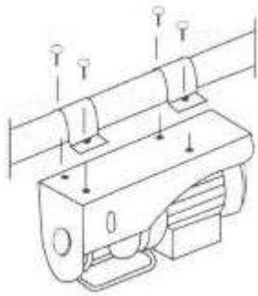
Рис.3 - Установка тали
