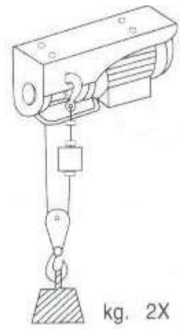
Рис.4 - Установка полиспаста
