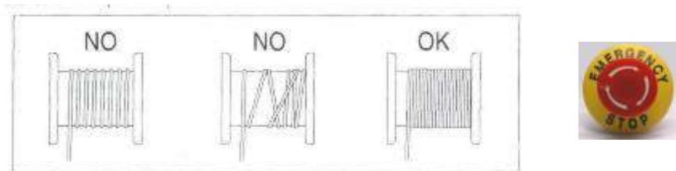
Рис.6 - Намотка троса на катушку
