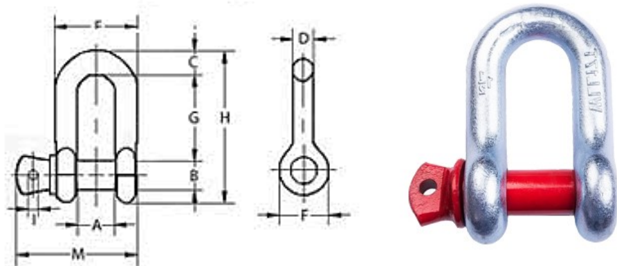
Рис.4 Схема скобы такелажной G210
