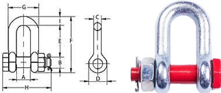
Рис.3 - Схема скобы такелажной G2150
