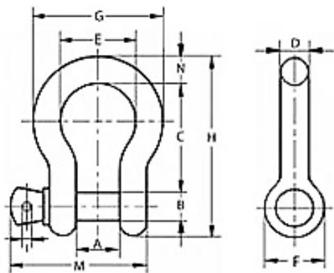
Рис.2 - Схема скобы такелажной G209
