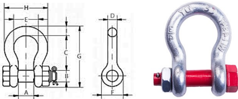
Рис.1 - Схема скобы такелажной G2130
