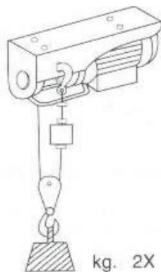
Рис.4 – Установка полиспаста
