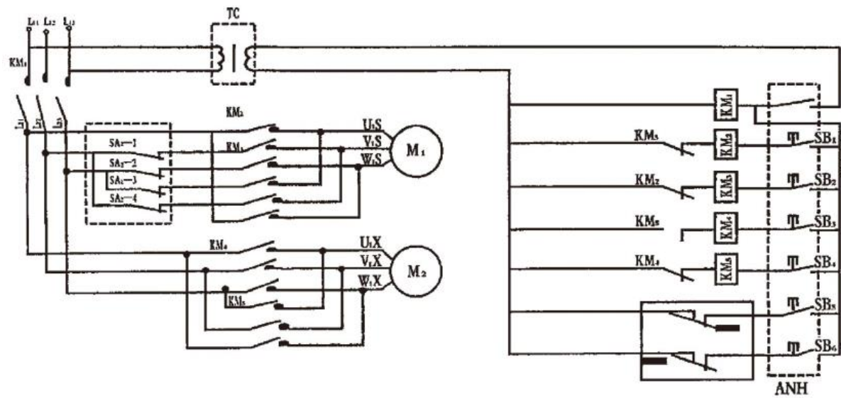
CDL 0,5-5T модель с понижающим трансформатором
