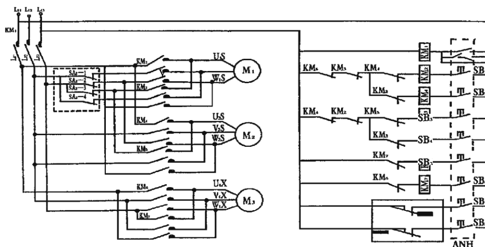
MDL 0,5-5T модель без понижающего трансформатора
