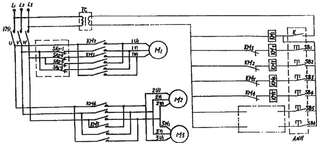
CDL 10 модель с понижающим трансформатором
