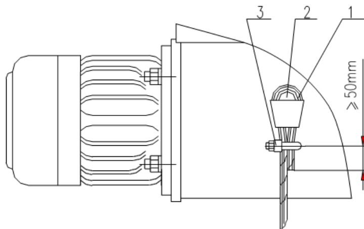
Схема установки каната
