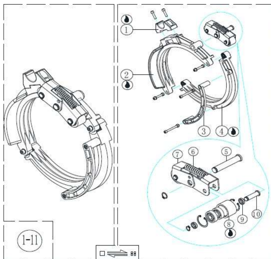
1-11 Канатоукладчик
