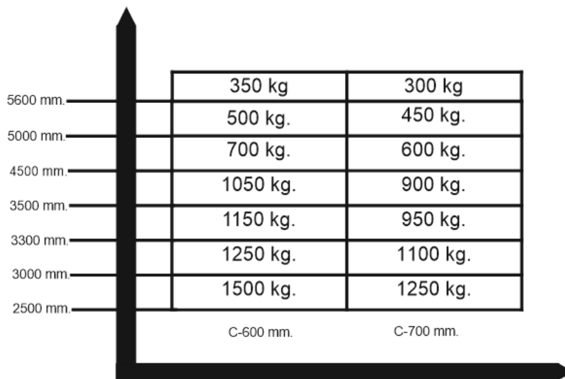
Рис.2 - График грузоподъемности C (mm) – центр загрузки вила (мм)
