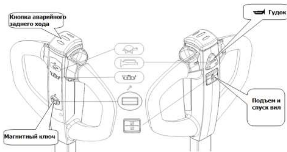
Рис. 6 – Рукоять управления
