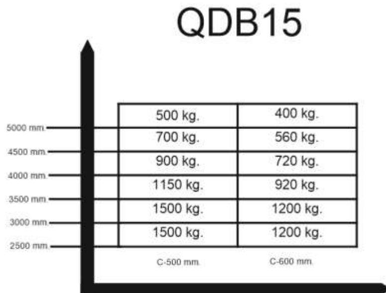
Рис. 3 – Кривая грузоподъемности
