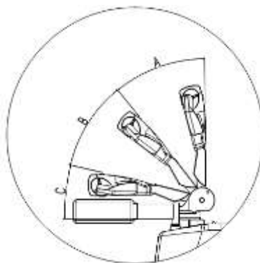
Рис. 7 – Положения рукояти
