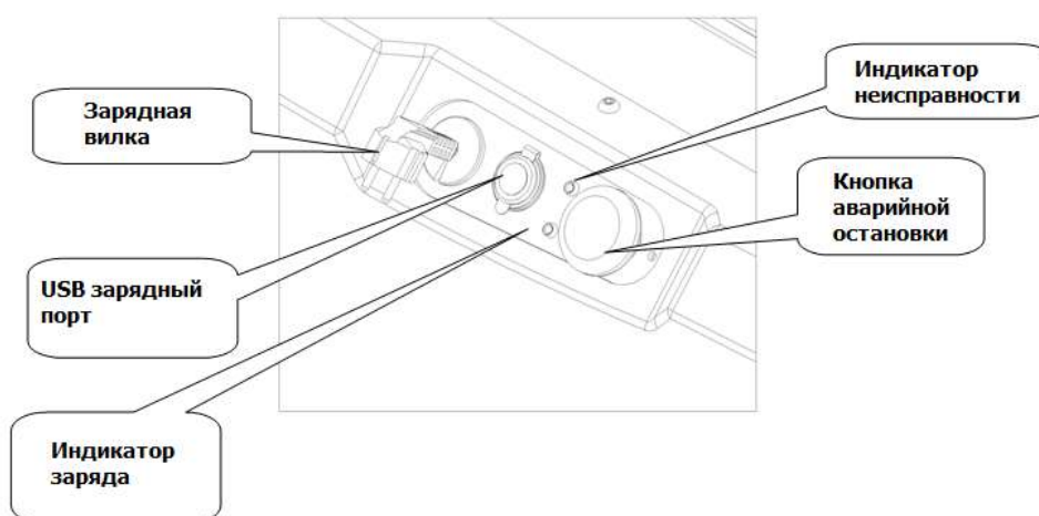
Рис. 4 – Элементы управления
