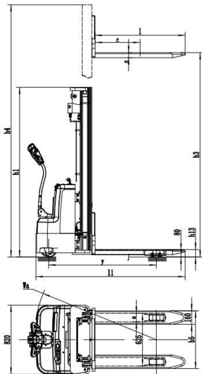
Рис.2 – Габаритные размеры
