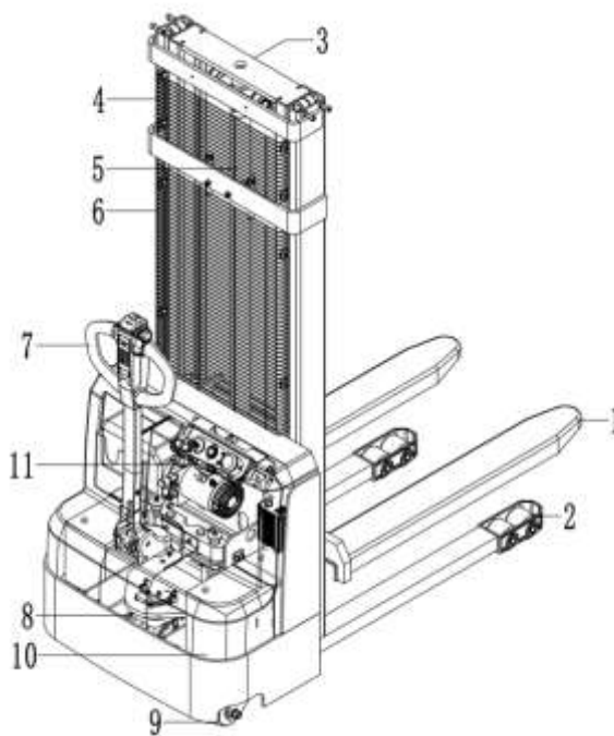
Рис. 1 – Устройство штабелера QDB
